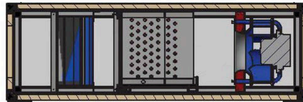
A-A (1:11)
